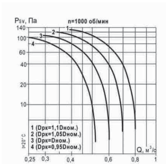
Аэродинамическая характеристика вентилятора ВКР №3,55
