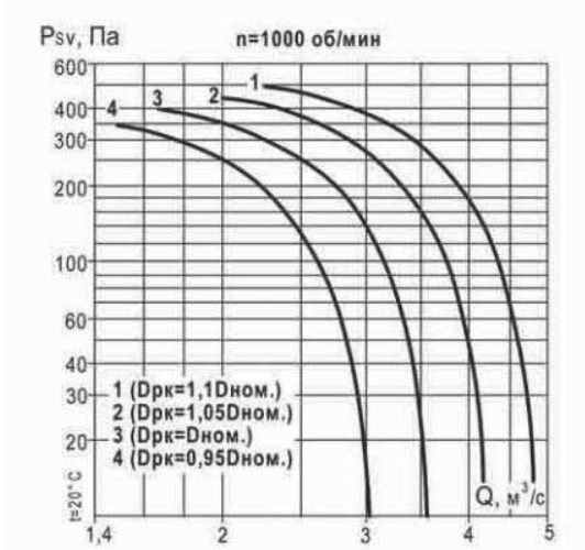
Аэродинамическая характеристика вентилятора № 6,3
