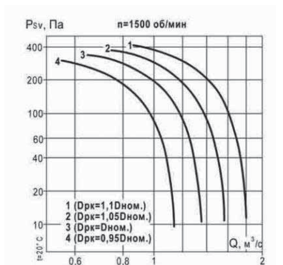
Аэродинамическая характеристика вентилятора ВКР №4
